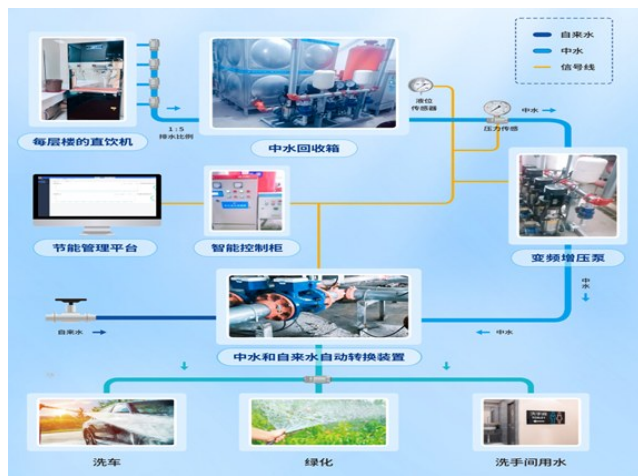
中水回收系统原理图
